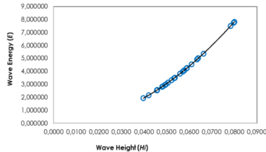
Fig 6: Relationship of parameter E with parameter H_i
